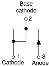
TO-220AC
